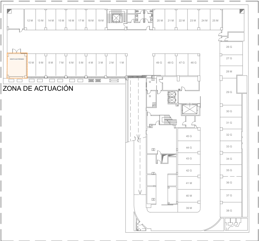
PLANTA SÓTANO -1. EDIF. CONDE DE PEÑÁLVER E:1/500
