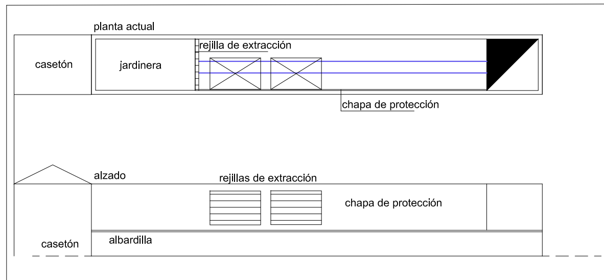
DETALLE UNIDADES EXTERIORES
