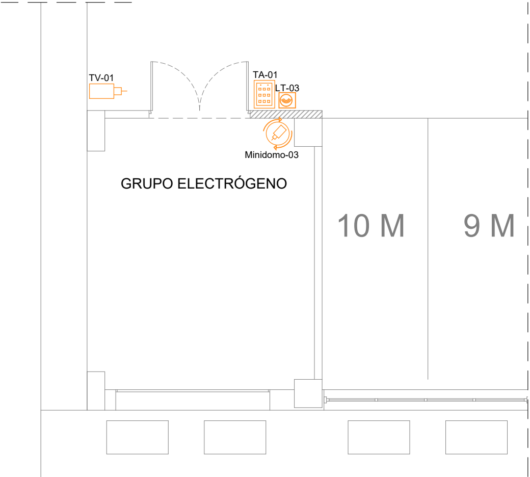
PLANTA SÓTANO -1
